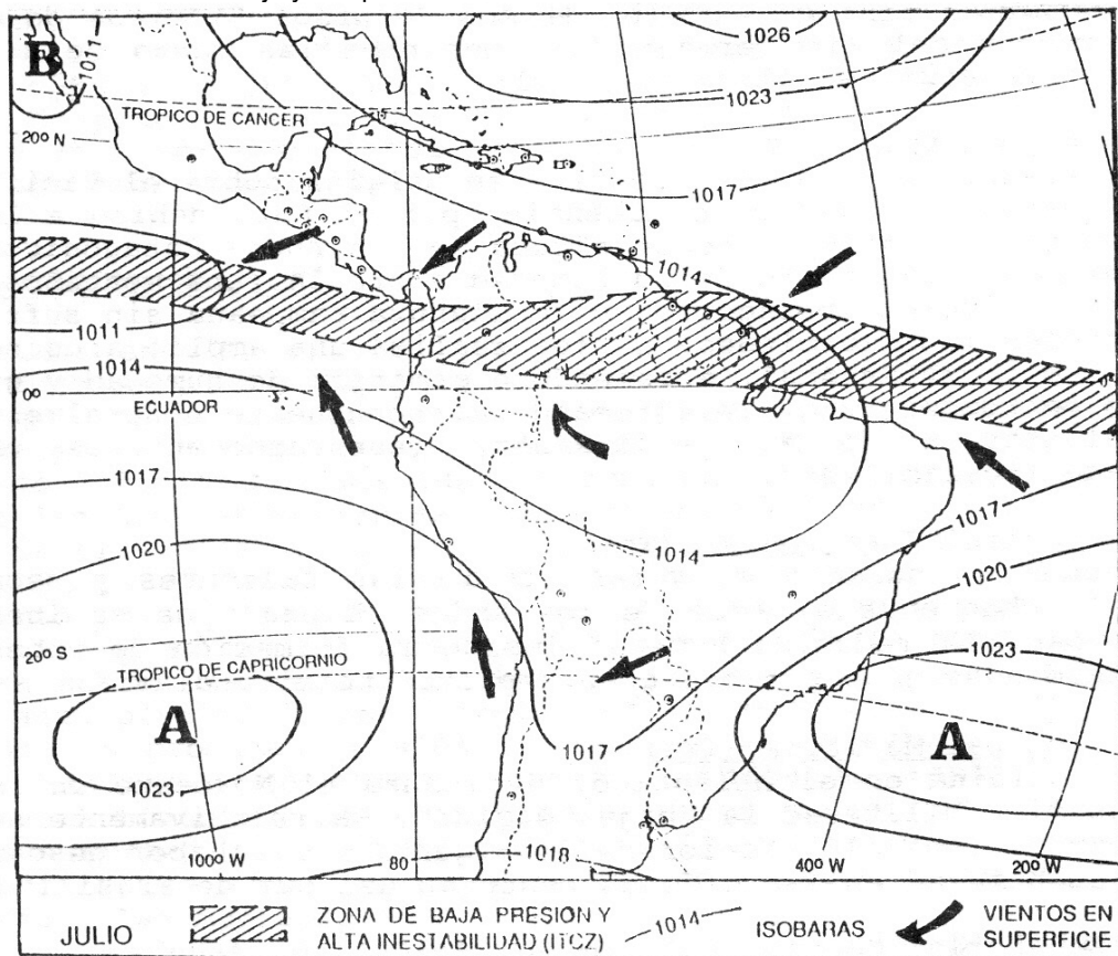
Mapa 3 – Situación atmosférica en Sudamérica en JULIO
