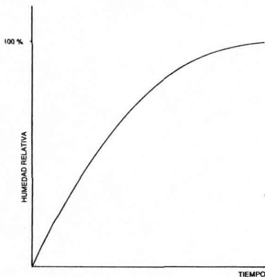
Fig. 1.- Si en recipiente con aire seco se agrega agua líquida, la humedad relativa del aire aumentará con el tiempo hasta alcanzar el 100 %
