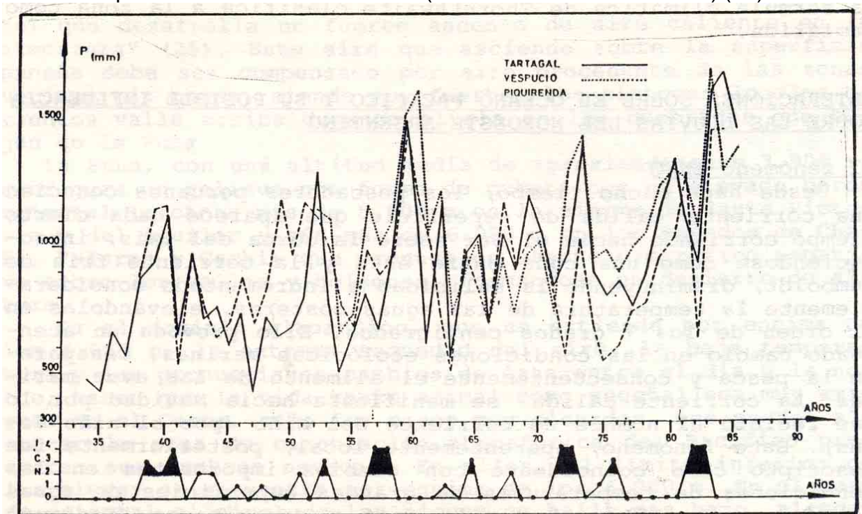
Fig. 6 - El fenómeno ENSO (El Niño/Southern Oscillation). Comparación de totales de precipitación anuales (P en mm) y la Intensidad de la Corriente del Niño (ICN).
