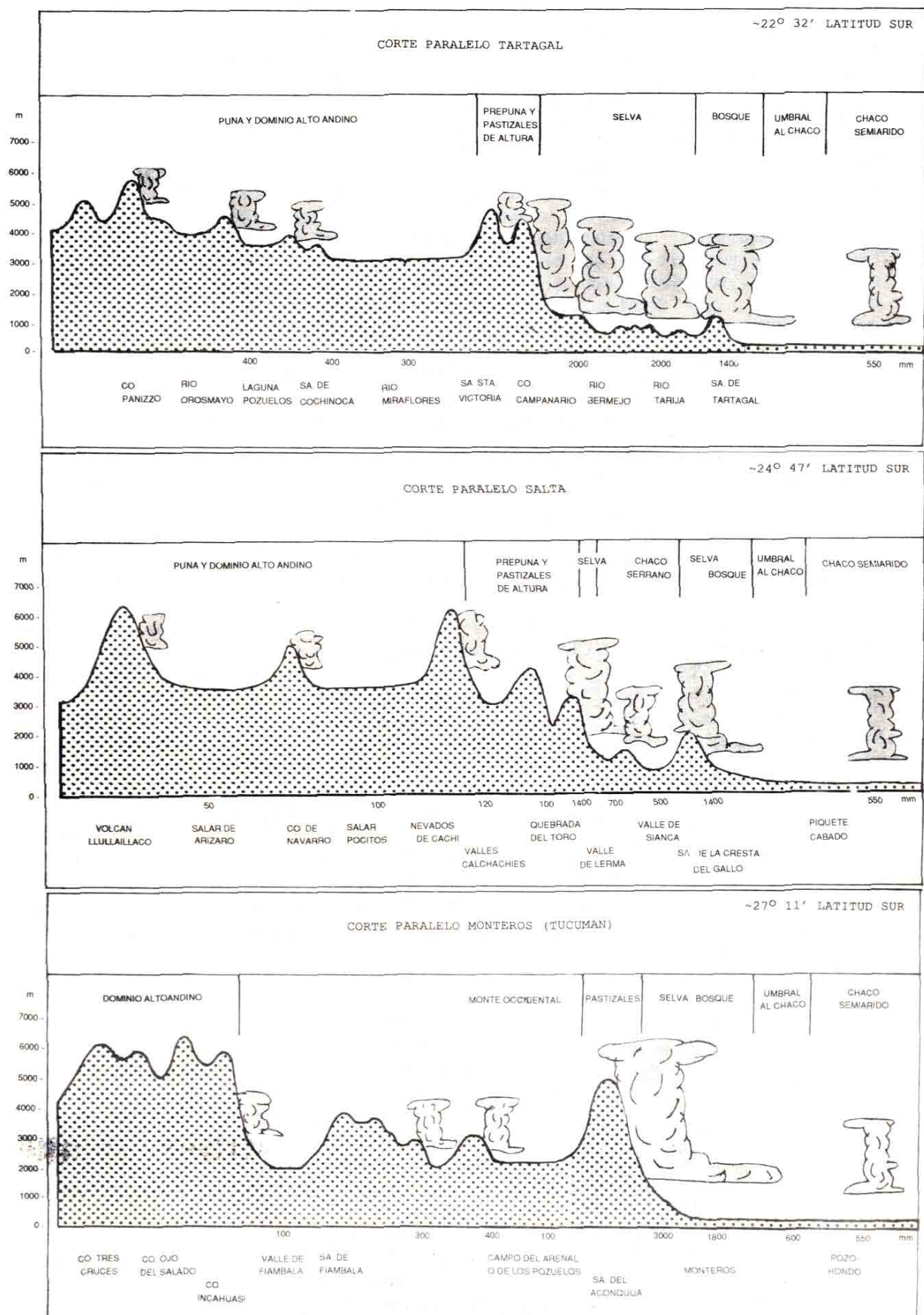
Fig. 4 - Distribución de las precipitaciones, fuertemente condicionada por el relieve, sobre tres paralelos (Tartagal, Salta y Monteros (Tucumán) y los ditintos biomas que en gran medida son determinados por ella.
