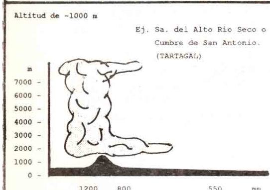
Fig. 3 - El efecto orográfico sobre las precipitaciones y su comportamiento con respecto a relieves de distinta altitud
