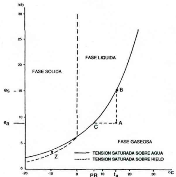
Fig. 2.- La tensión de vapor del aire saturado con vapor de agua aumenta cuando aumenta la temperatura del aire. ( t_a = temperatura actual del aire, PR = temperatura del punto de rocío, e_a = tensión de vapor actual, e_s = tensión de vapor de saturación).
