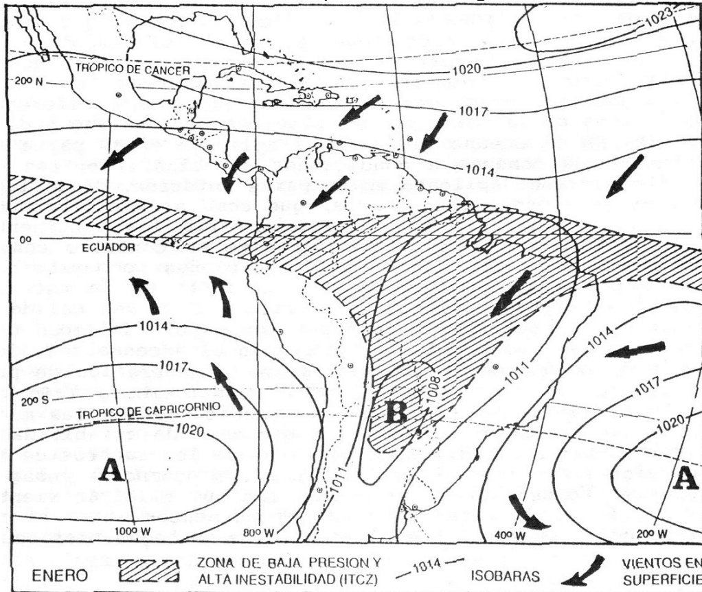
Mapa 3 – Situación atmosférica en ENERO. Isobaras y vientos en superficie; ubicación de la ITCZ; centros de baja y alta presión.
